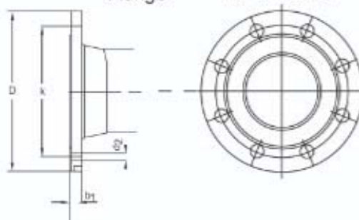
Flange
