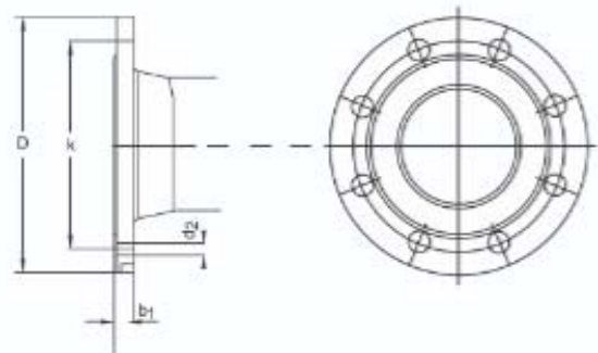
Flange
