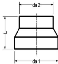
تبدیل هم مرکز پلی اتیلن مطابق استاندارد ISIRI ۱۴۴۲۷/PE۱۰۰
