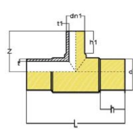
سه راهی پلی اتیلن مطابق استاندارد PE100/ISIRI14427
