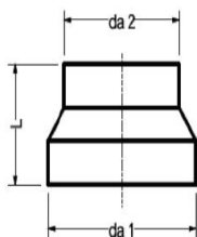
تبدیل هم مرکز پلی اتیلن مطابق استاندارد PE100/ISIRI14427
